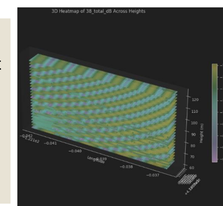
Fig. 14. RSRP Fading
